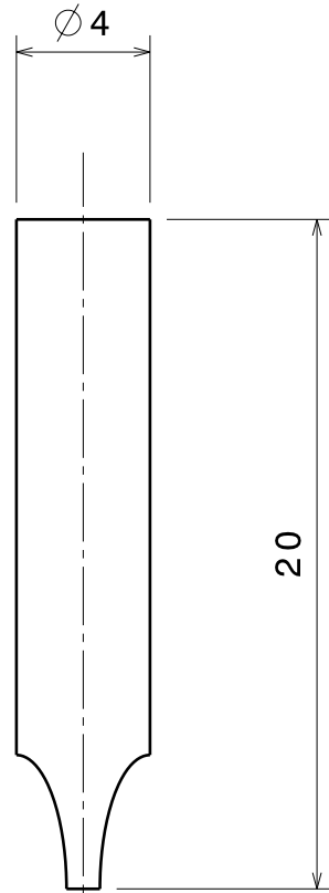
Bottom view Scale: 4:1
